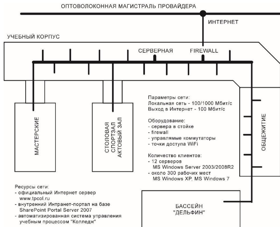
Рисунок 3. Схема корпоративной сети колледжа
